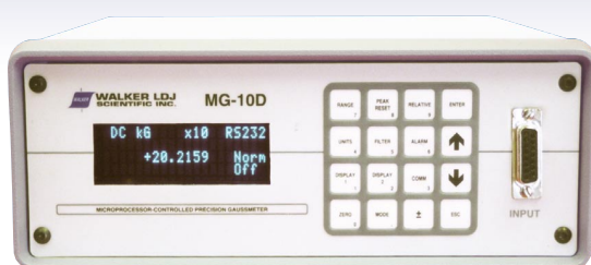
MG-10D GAUSSMETER
